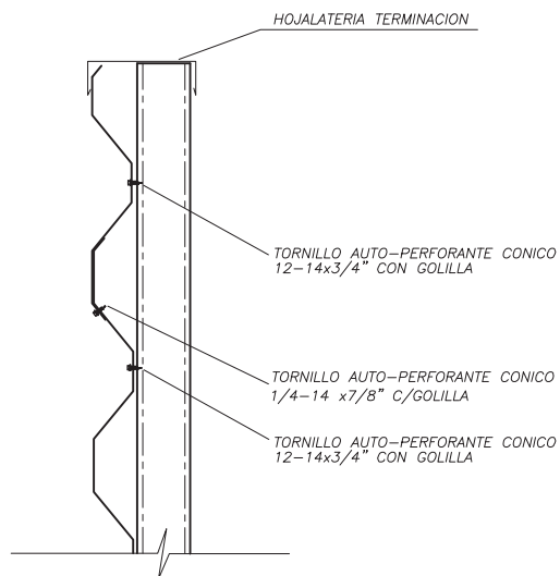
DETALLE FIJACION REVESTIMIENTO HORIZONTAL
