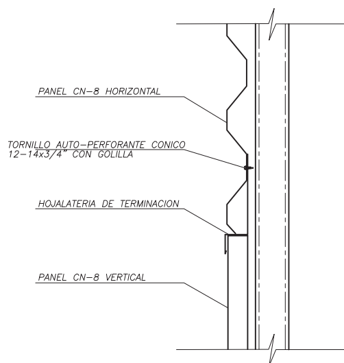
DETALLE REVESTIMIENTO HORIZONTAL Y VERTICAL
