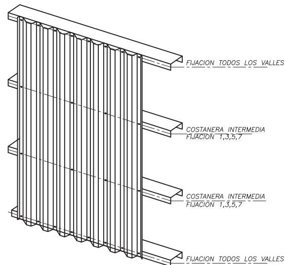
SISTEMA DE FIJACION
