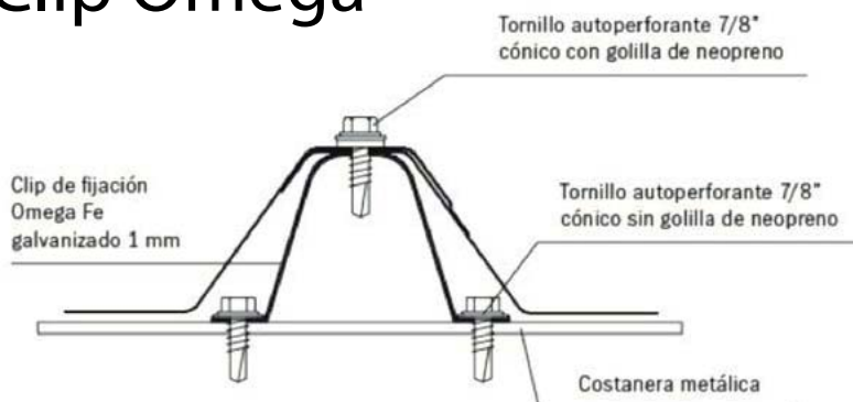
CLIP OMEGA (usa 3 tornillos)
