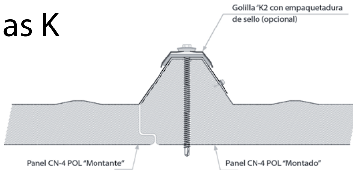
CORTE TÍPICO EN FIJACION DE PANEL CN-4 POL
